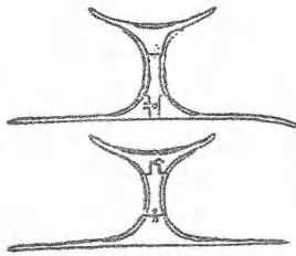
مساند رأس مشكلة من ثلاثة اجزاء ومعشقة بوصلة النقر واللسان المدعمة بالخوابير الخشبية، دولة قديمة
